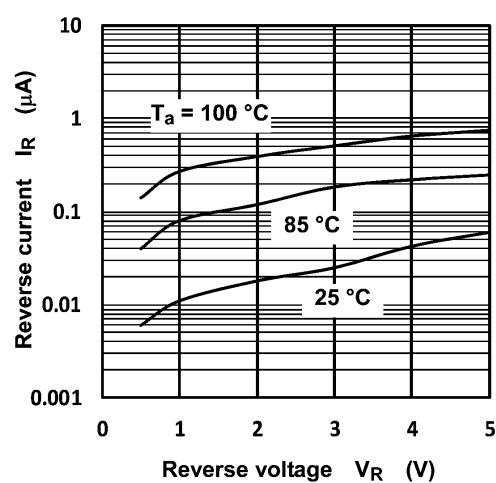
Fig. 9.2 I_R - V_R
