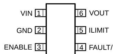
SOT 23-6 (M6)
