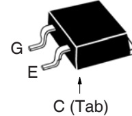
TO-268HV (IXBT)
