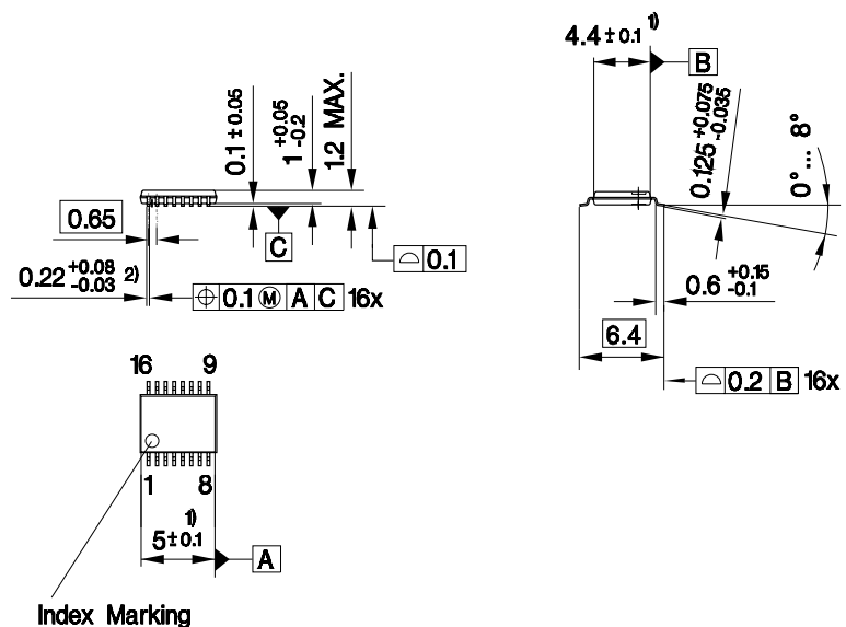
P-TSSOP-16-1
