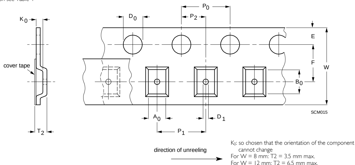
Fig. 4 Blister tape
