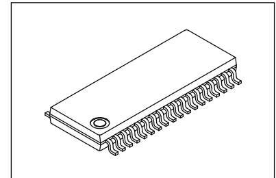
SSOP36J (275mil)
