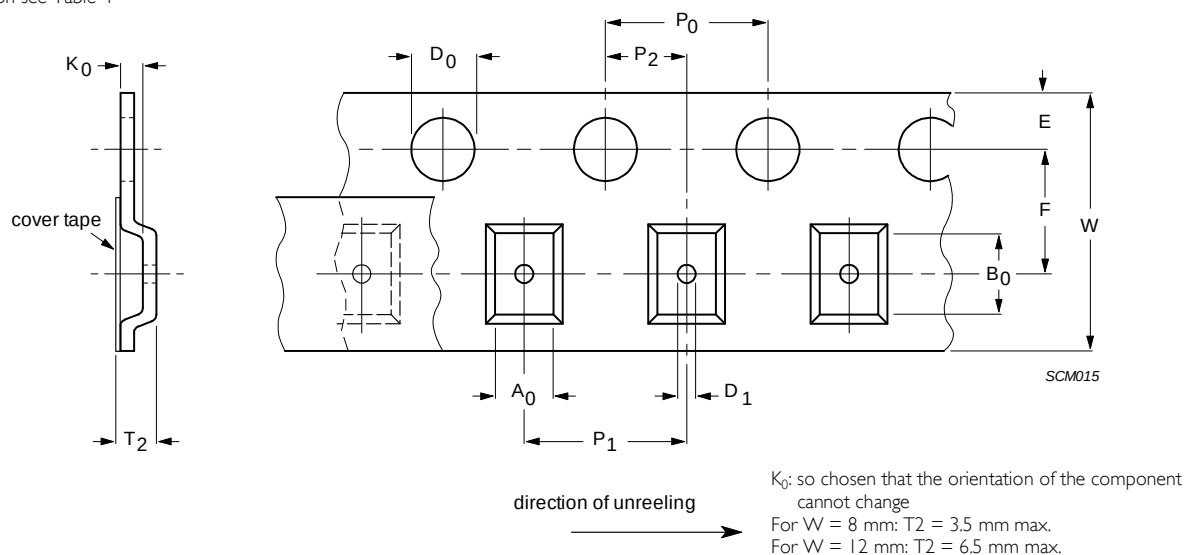
Fig. 4 Blister tape
