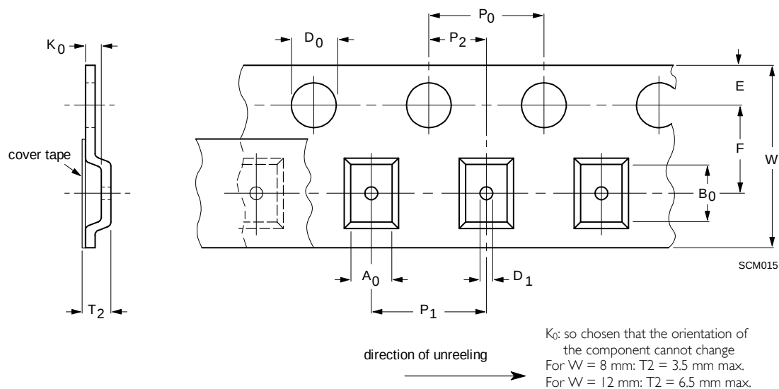
Fig. 4 Blister tape
