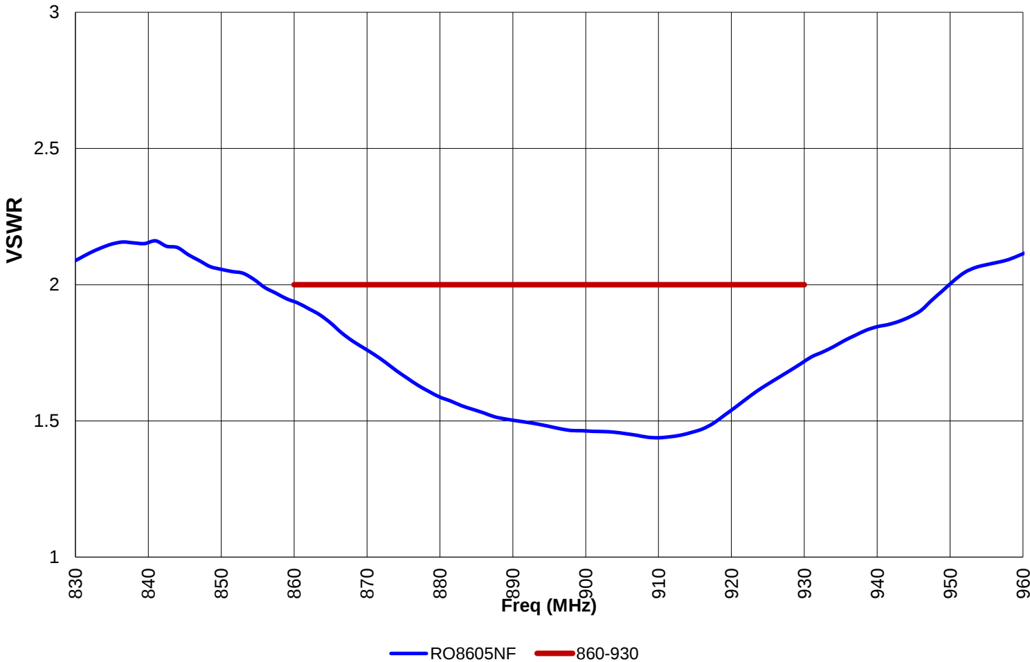
S11 Parameter
