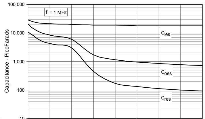
Fig. 8. Capacitance
