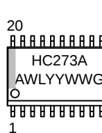
SOIC-20
