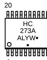
TSSOP-20
