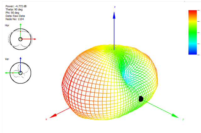
2150 MHz
