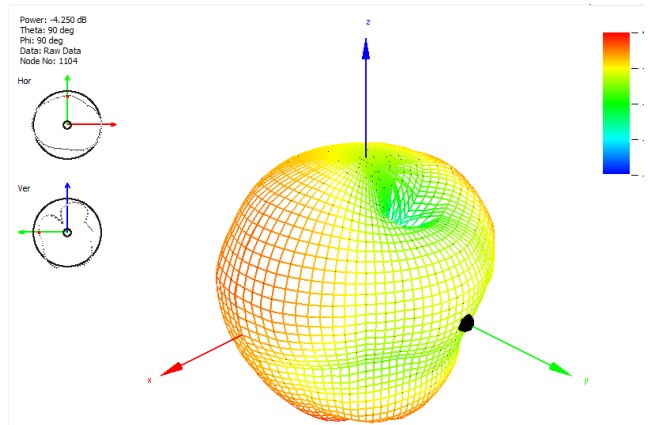
2450 MHz
