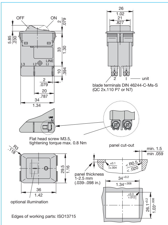
Dimensions 3130-F120-...
