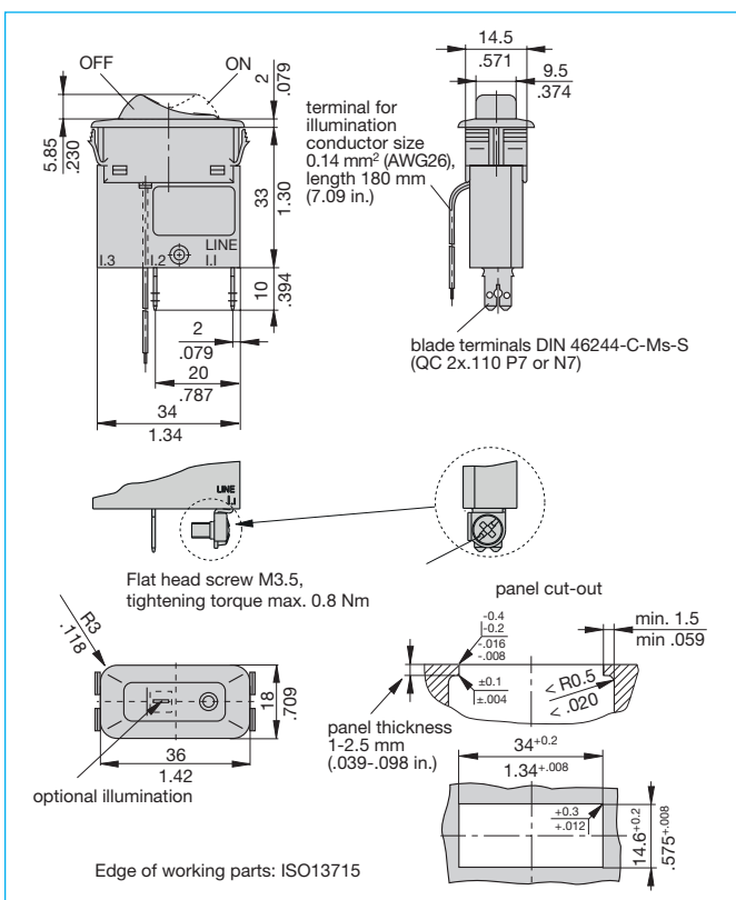
Dimensions 3130-F110-...
