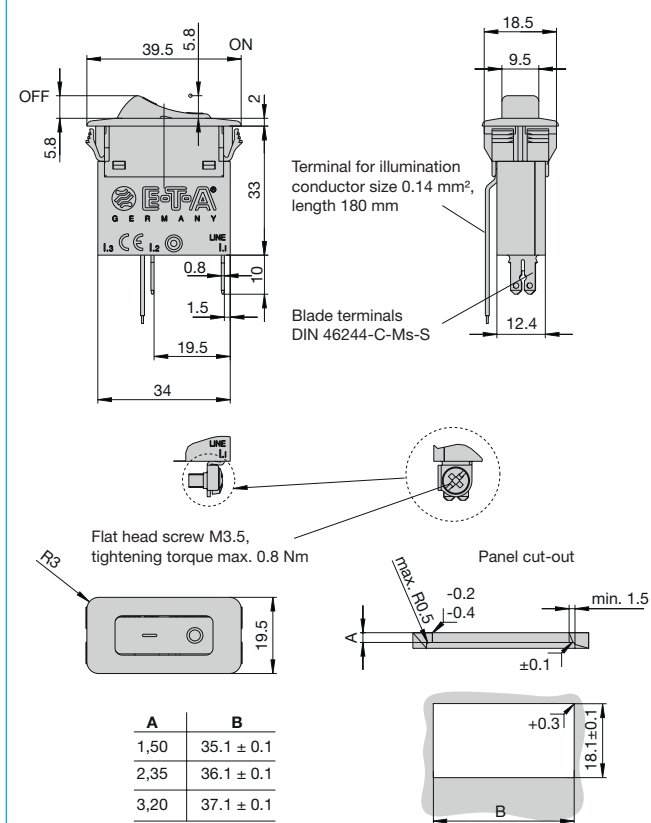
Dimensions 3130-F120-...
