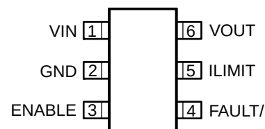
SOT 23-6 (M6)
