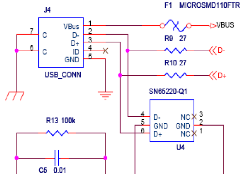
Figure 4-5. USB Mini Port Schematic
