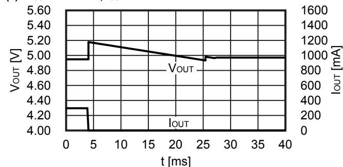
(2) f_{OSC} = 1.2\text{ MHz} , I_{OUT} = 300\text{ mA} \rightarrow 0.1\text{ mA} S-8365AABBA
