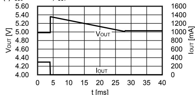
(4) f_{OSC} = 600\text{ kHz} , I_{OUT} = 300\text{ mA} \rightarrow 0.1\text{ mA} S-8365ABBBA
