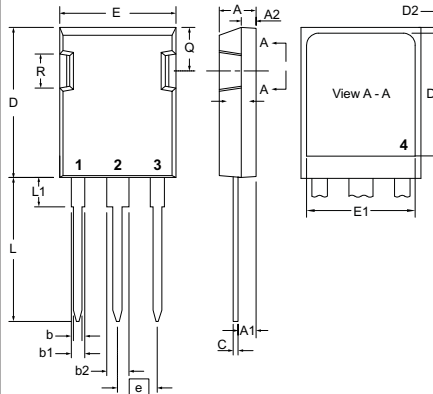
X015a PLUS247™
