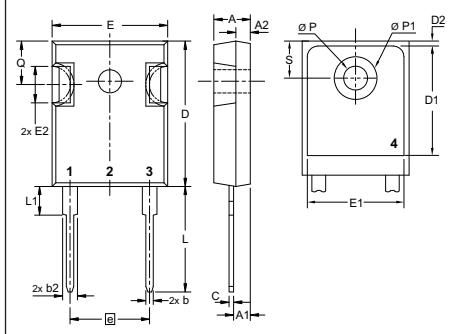
X014b TO-247 AD
