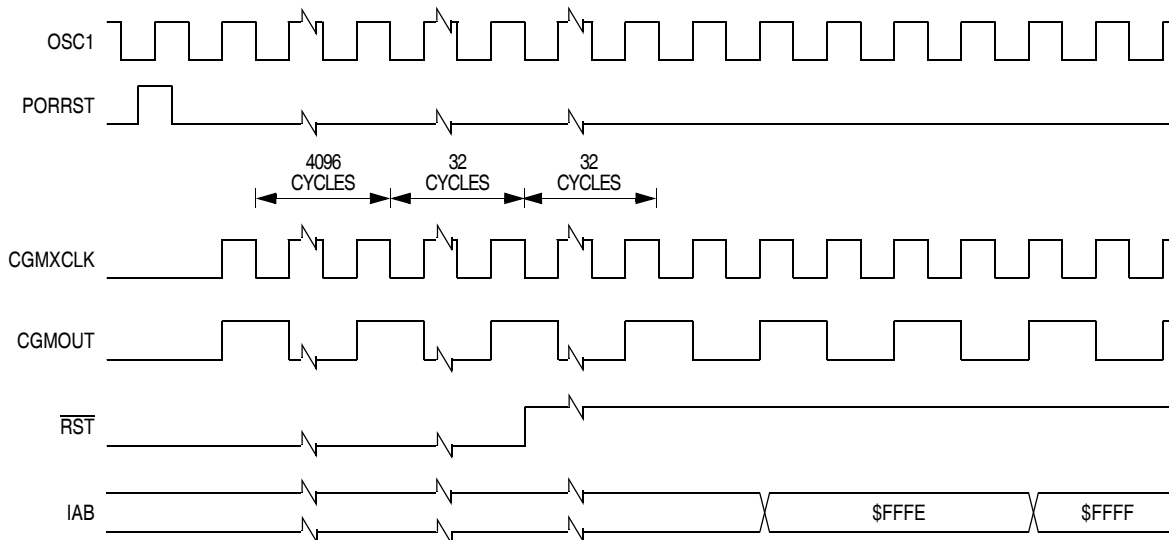
Figure 15-7. POR Recovery
