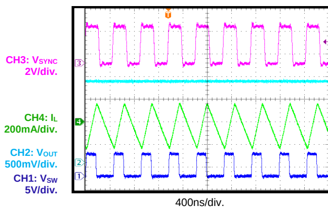
SYNC Input
