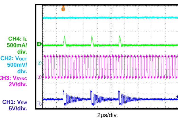
SYNC Input
