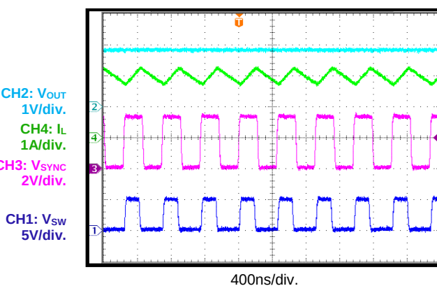
SYNC Input
