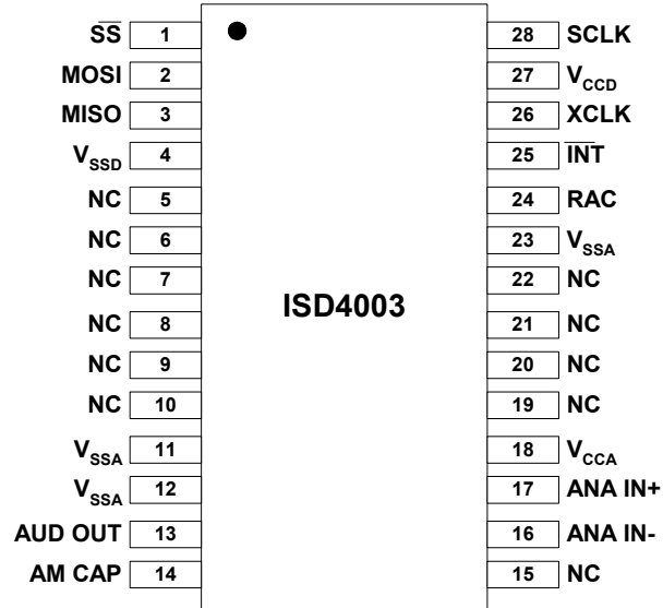
SOIC / PDIP
