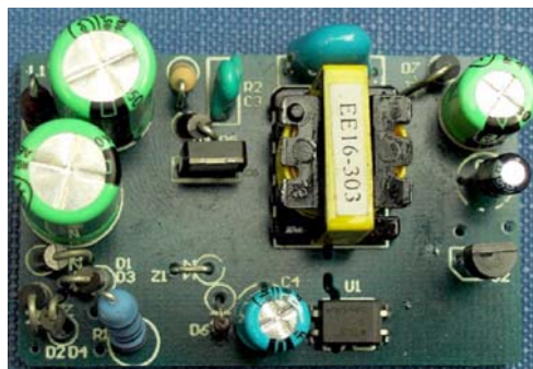
STEVAL-ISB001V1
