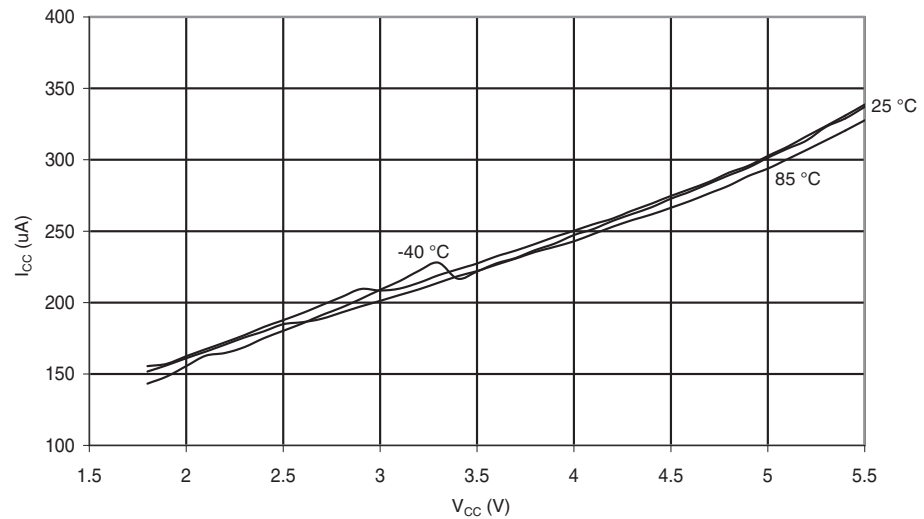
Figure 30-131. ADC Current vs. V CC (AREF = AV CC ).
