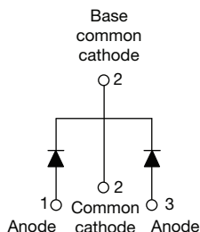
VS-20CTQ150-1-M3
