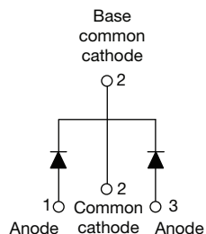
VS-20CTQ150S-M3
